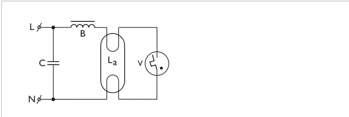
EM BALLAST
